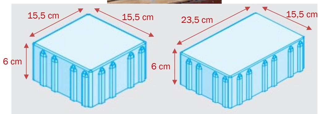
Figure 2 - Revêtement constitué et géométrie des pavés
