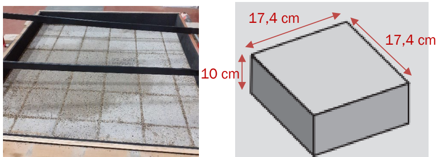
Figure 2 - Revêtement constitué et géométrie des pavés
