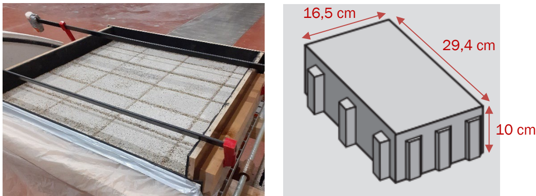
Figure 2 - Revêtement constitué et géométrie des pavés
