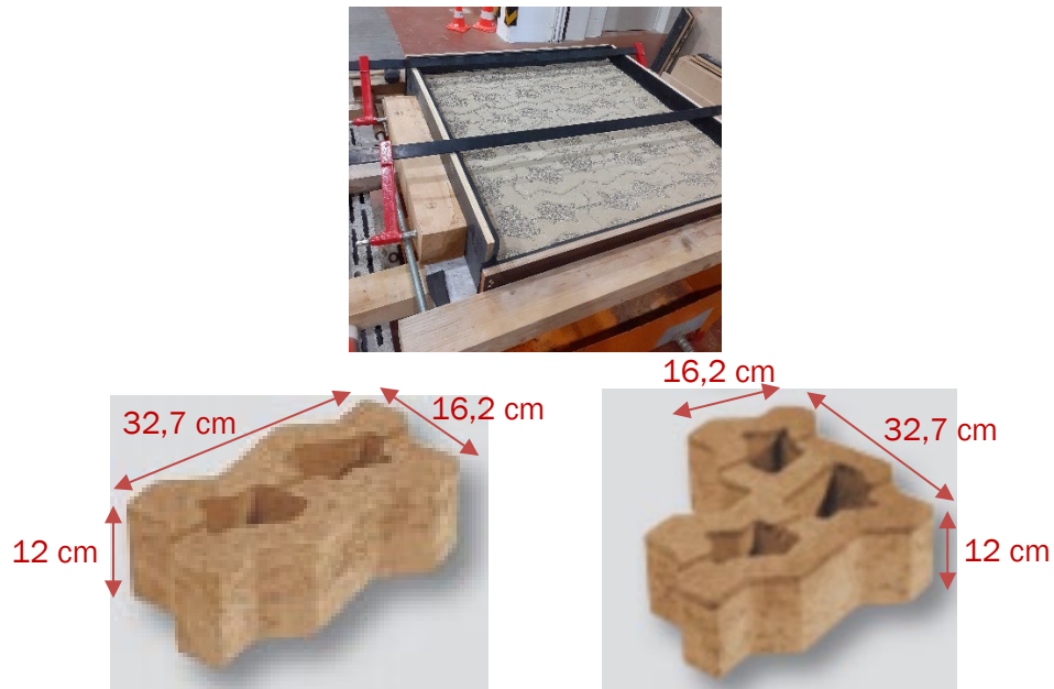
Figure 2 - Revêtement constitué et géométrie des pavés
