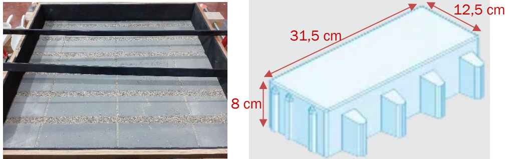
Figure 2 – Revêtement constitué et géométrie des pavés
